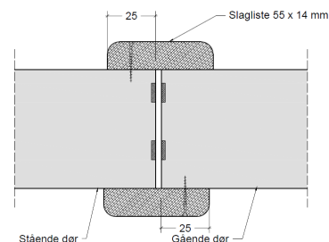
BD60 dobbeltdør
