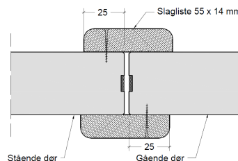
BD30 dobbeltdør
