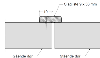
Uklassificeret dobbeltdør
