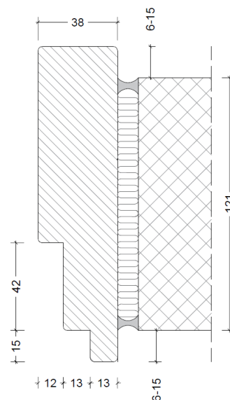
Karm med fremspring
