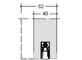
Hæve/sænke bundtætningsskinne
