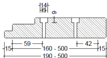
Illustration 4: Forboring af karm fra 190 mm
