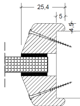
40mm m. F30 glas fig. 2
