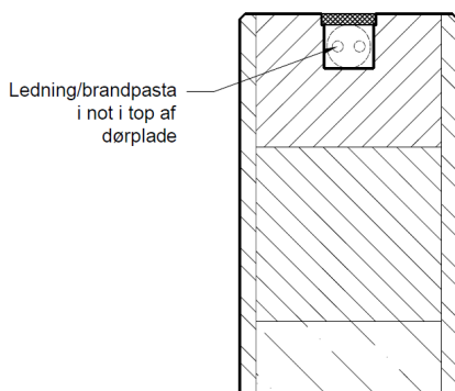
Lodret snit
