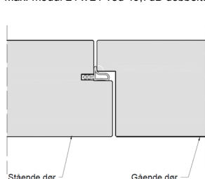
CS 200 dobbeltdør
