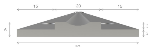
Snit af bundskinne
