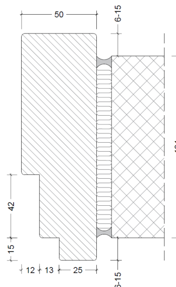
50 mm karm med fremspring (kun 49,7dB)
