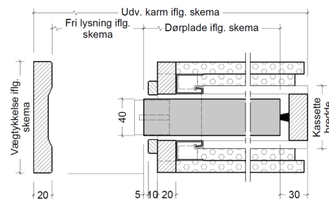
Væg m. 2+2 lag gips
