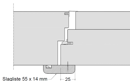
BD30/49,7dB dobbeltdør
