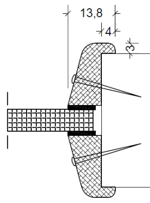
40mm m. uklassificeret glas fig. 1
