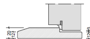
Træbund 62 mm dør
