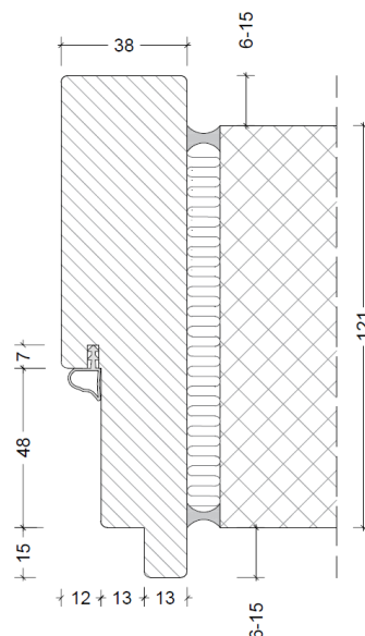
Karm med fremspring og tætningsliste
