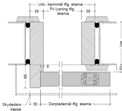
Blændkarm type 3 med anslag
