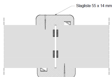
BD30/35dB + BD30/40dB + BD60/35 BD60/40dB dobbeltdør
