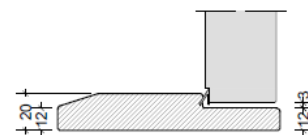
Træbund 40 mm lyddør
