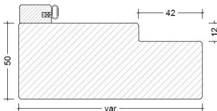
Standard karm til 49,7dB
