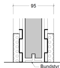
Bund af skydedørselement
